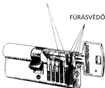
Fúrás elleni védelem fúrásvédő csappal
